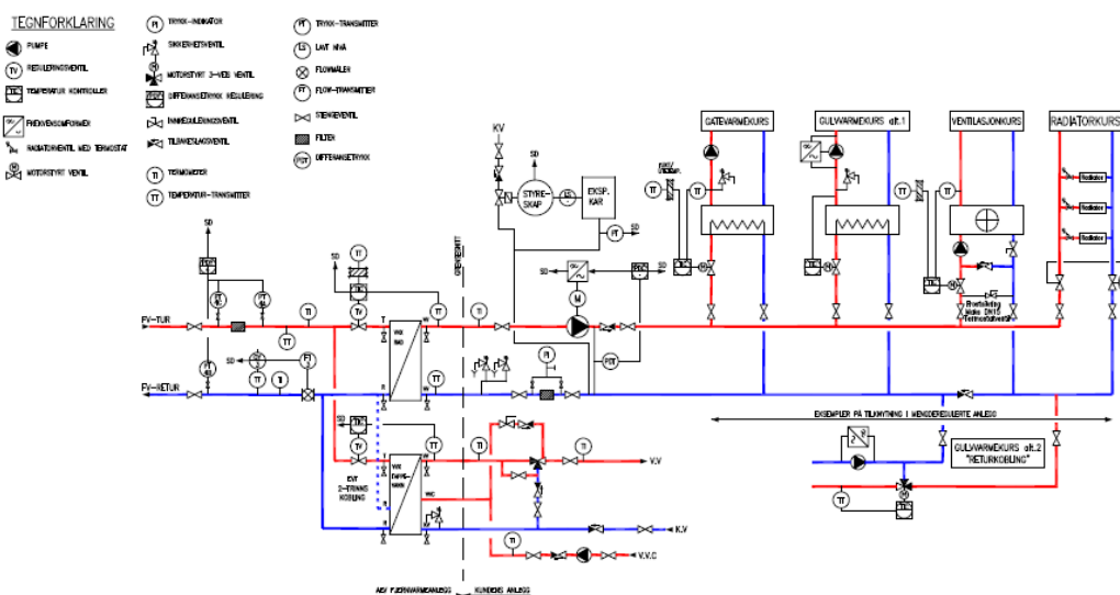
Figur 3: Direkte tappevannsveksling
