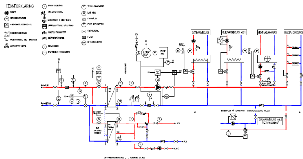
Figur 3: Direkte tappevannsveksling
