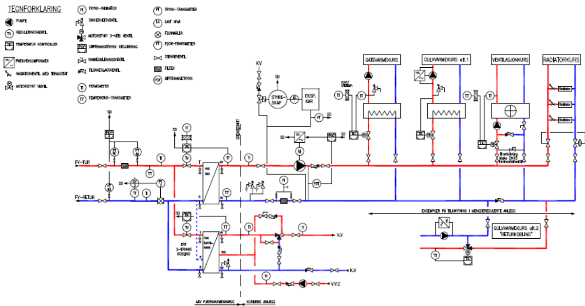
Figur 2: Systemskisse. Teknisk utforming samt ansvarsgrenser for investering, drift og vedlikehold.
