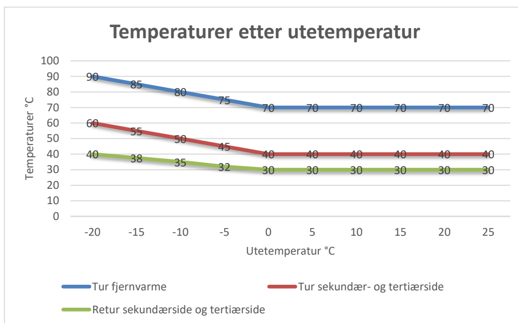
Figur 1: Eksempel på variasjon av temperaturen på tur fjernvarme, tur- og retur på sekundærsiden avhengig av utetemperatur.
